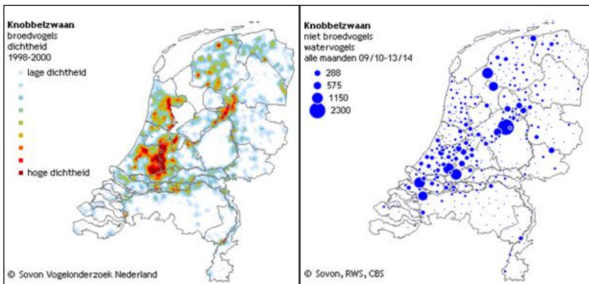
Abbeelding 2: Links: Verspreiding (relatieve dichtheid) van de knobbelzwaan als broedvogel in Nederland. Weergegeven is de relatieve dichtheid in 1998-2000. Bron: Sovon (2002). Rechts: Verspreiding (gemiddeld aantal per hoofdtelgebied) van de knobbelzwaan in Nederland. Weergegeven is het gemiddelde aantal per (hoofd)telgebied in 2009/10-2013/14. Veel grote wateren worden jaarrond geteld; de overige gebieden doorgaans alleen in september-april. Bron: Netwerk Ecologische Monitoring (NEM), Meetnet Watervogels.
